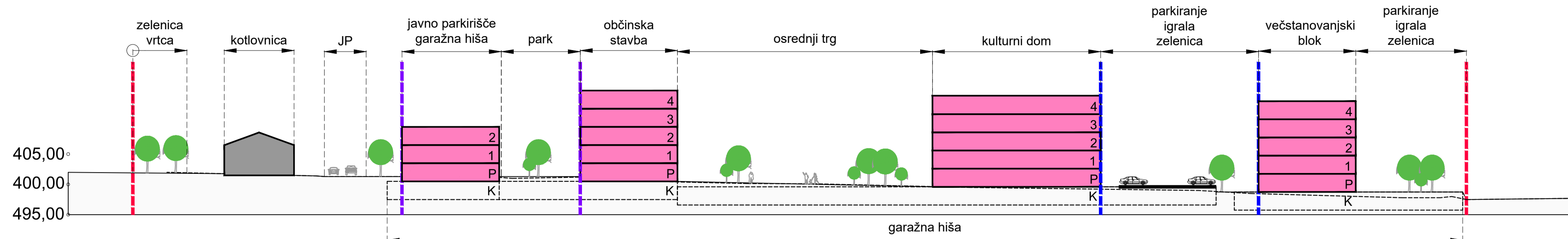
PREREZ A - A, M 1:500
